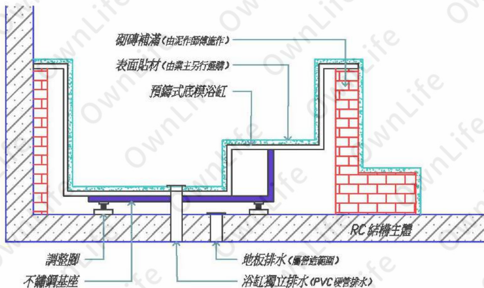
預鑄式底模結構剖面圖
