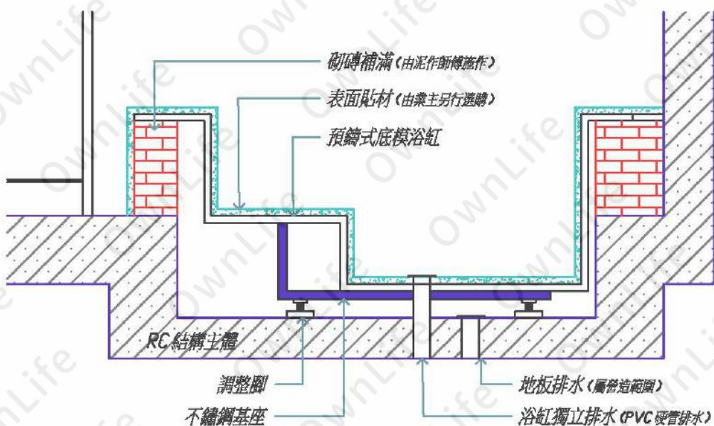
降板預鑄式底模結構剖面圖
