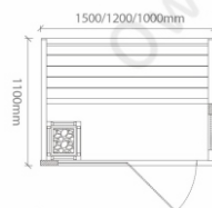
OW-B2521-SW 1500*1100*1900mm 1200*1100*1900mm 1000*1100*1900mm
