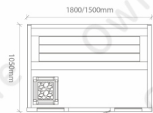
OW-6051-SW 1500*1050*1900mm 1800*1050*1900mm
