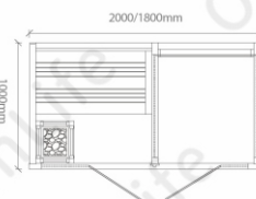
OW-5041-SW 2000*1000*2100mm 1800*1000*2100mm
